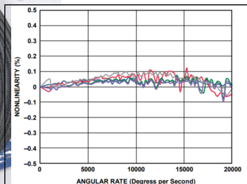
非线性度
